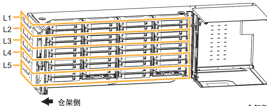
左侧剖面图
